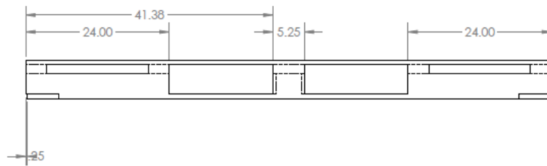
Abbildung 2: Abmessungen auf der langen Seite der Palette
